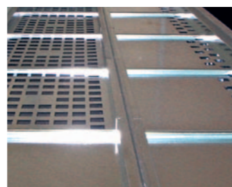
Paint-stop filter trays for air evenness in the booth box. Bandejas selectoras del flujo de aire en el basamento.
